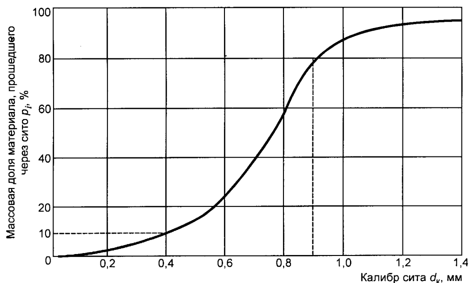
Рисунок А.1 — График ситового анализа материала
