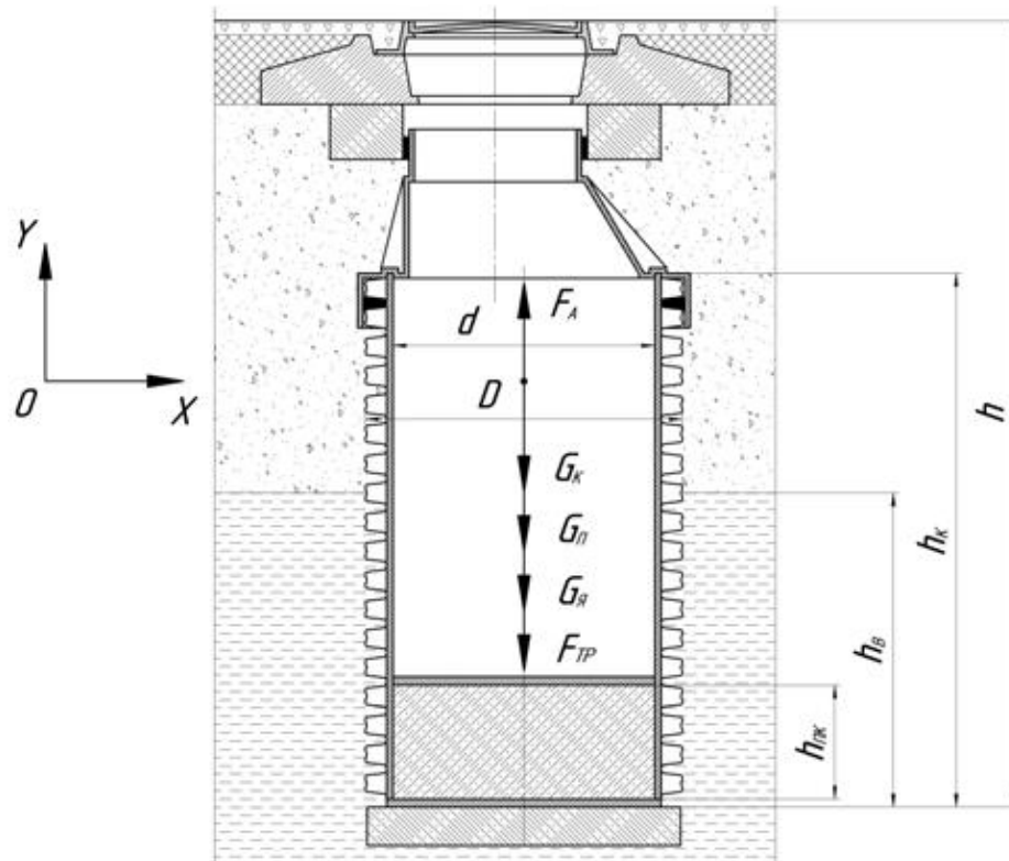
Схема действующих сил на колодец:
