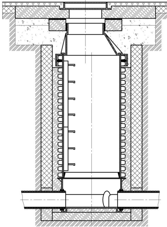
Рисунок 44 – Восстановленный кирпичный колодец
