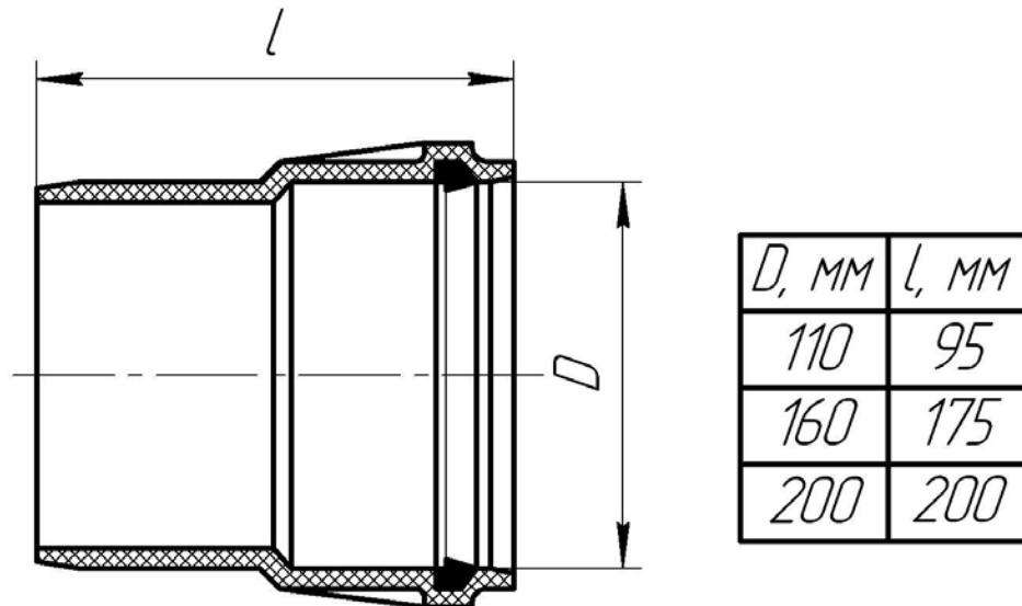
Рисунок 39 – Уплотнительная манжета и её типоразмеры.
