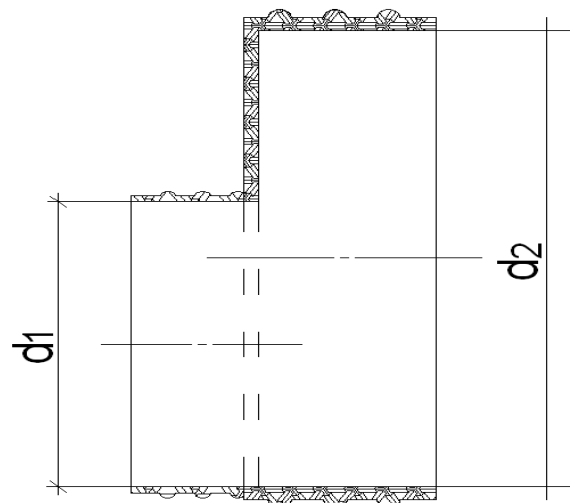
Рисунок 42 – Эксцентрический переход
