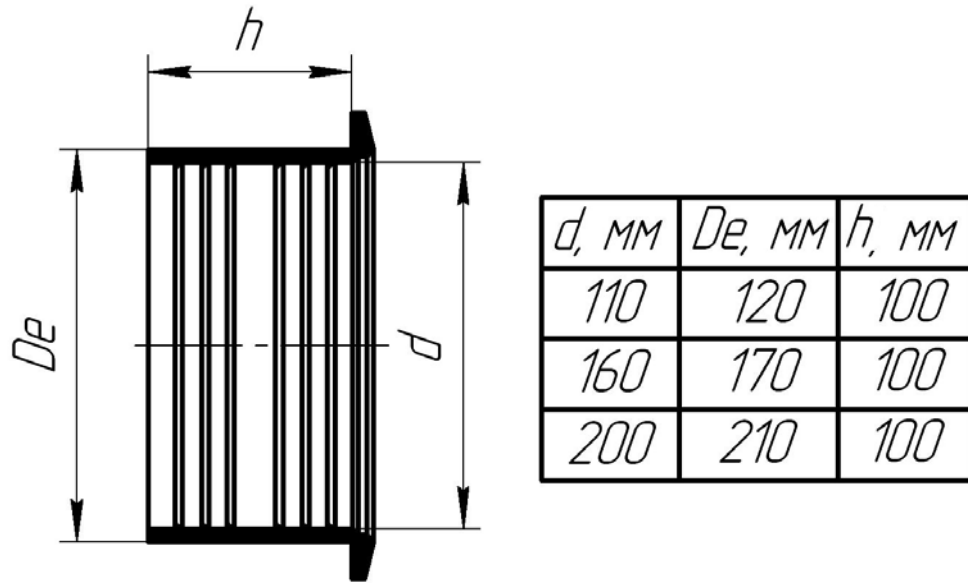
Рисунок 39 – Уплотнительная манжета и её типоразмеры.
