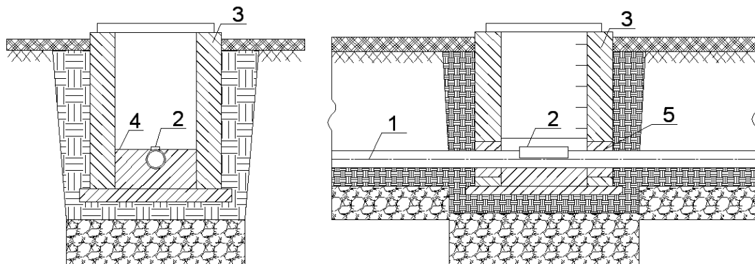
1 – труба; 2 – ревизия; 3 – колодец; 4 - дно колодца (бетон); 5 - эластичное уплотнение. Рисунок 43
